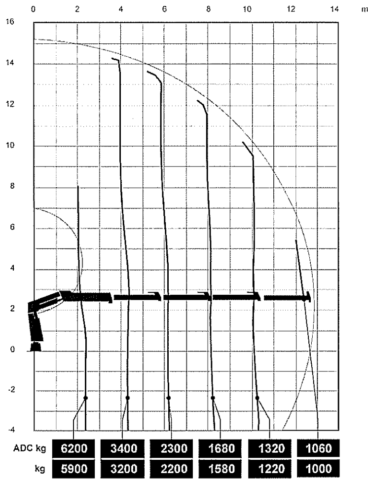
Belastungsdiagramm
